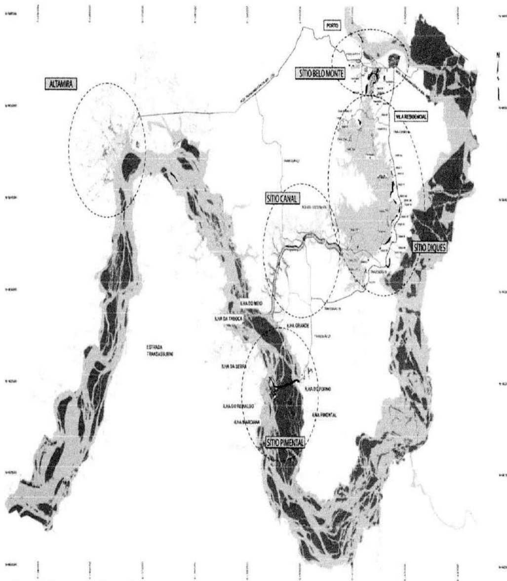
Figura 1 - Layout Geral UHE Belo Monte
